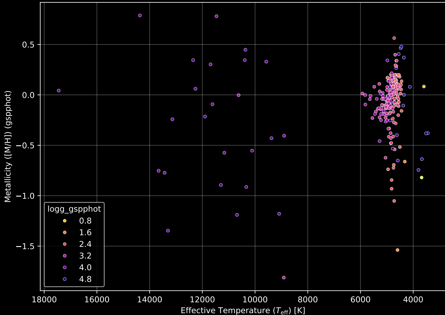
APOGEE DR17 Field: [090+08] Stellar Population Parameters (n= 239)
